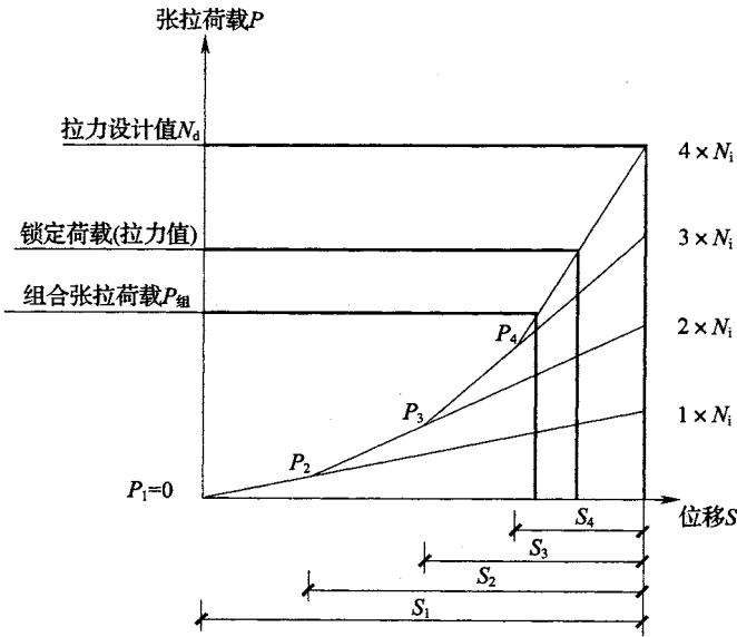
图 C. 0. 2-2 张拉管理图
