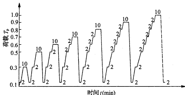
图 H. 0.1 锚杆基本试验多循环张拉试验的加荷模式(黏性土中)
