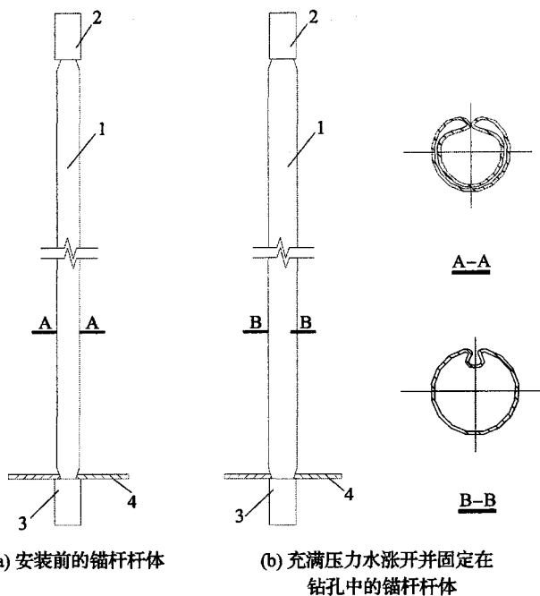
图 A.0.5 水胀式锚杆结构图
